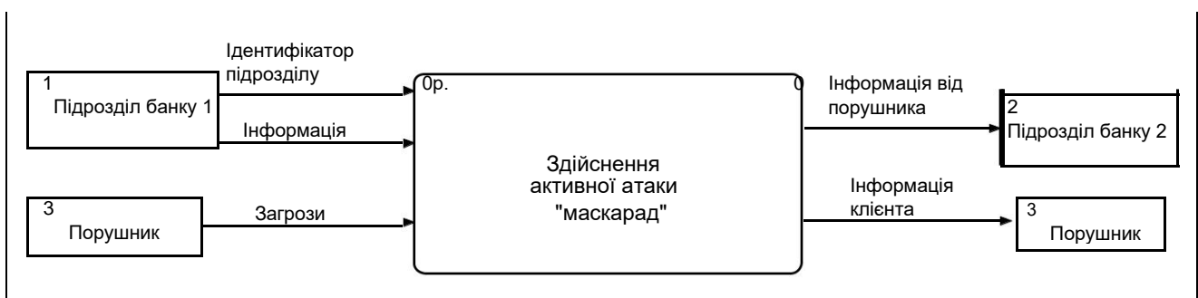
Рис. 1.15. Модель активних атак "маскарад"
