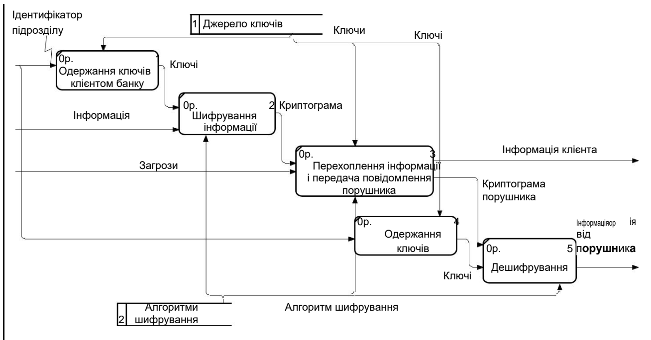
Рис. 1.16. Декомпозиція моделі активної атаки "маскарад"
