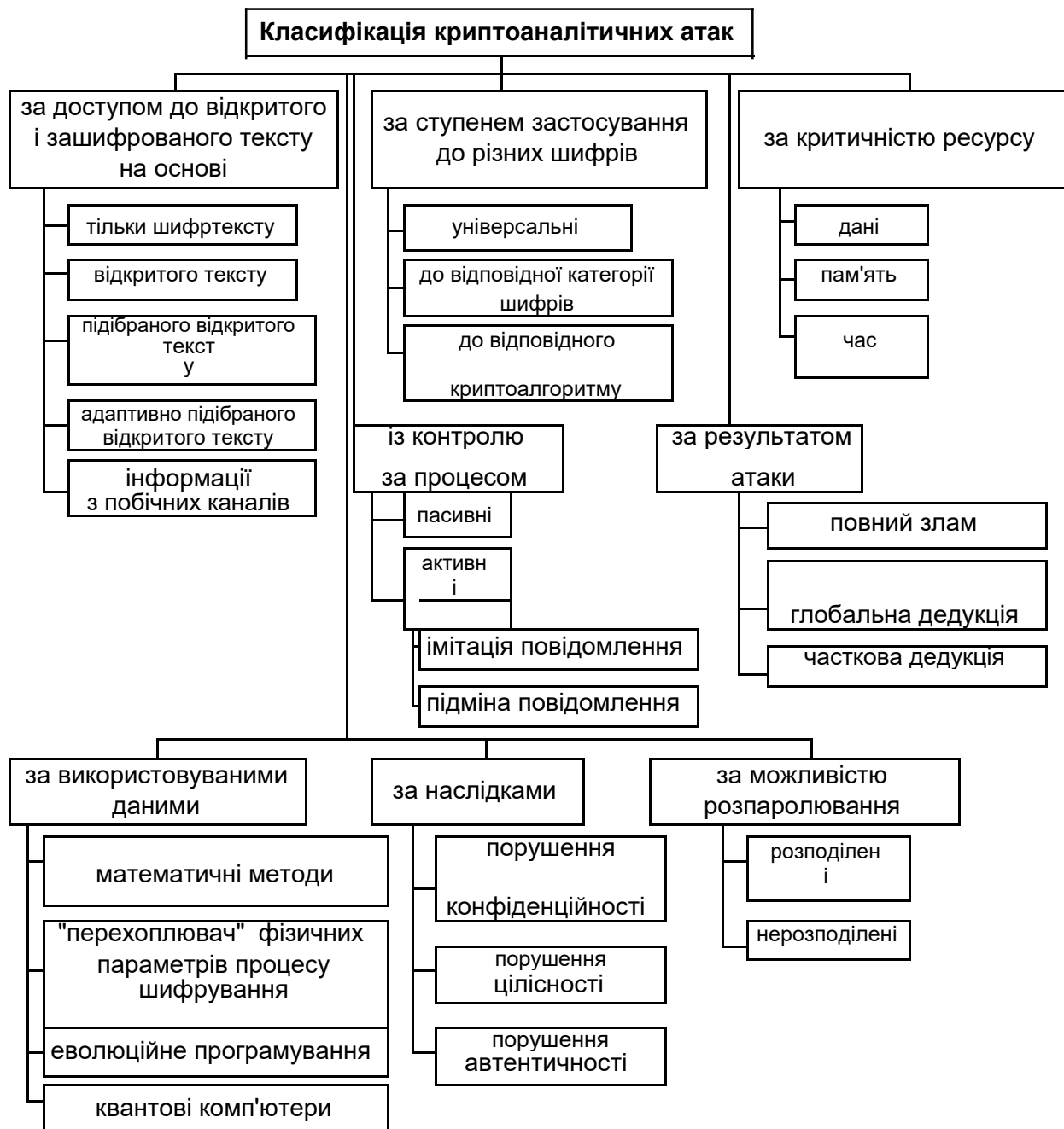
Рис. 1.3. Класифікація криптографічних атак
