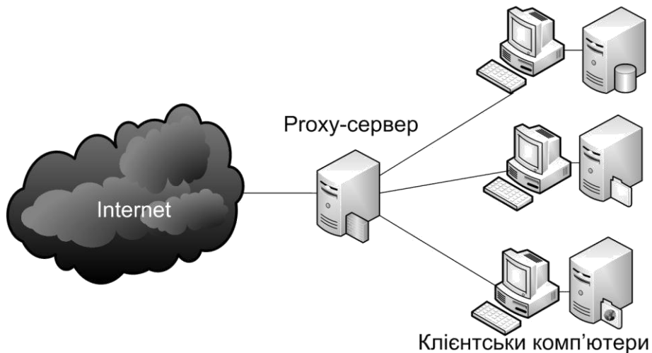
Рис. 2.6. Proxy-сервер
