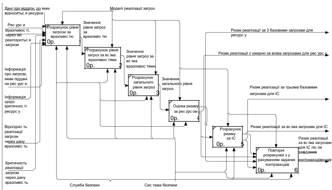
Рис. 1.18. Декомпозиція моделі оцінювання ризику реалізації загроз
