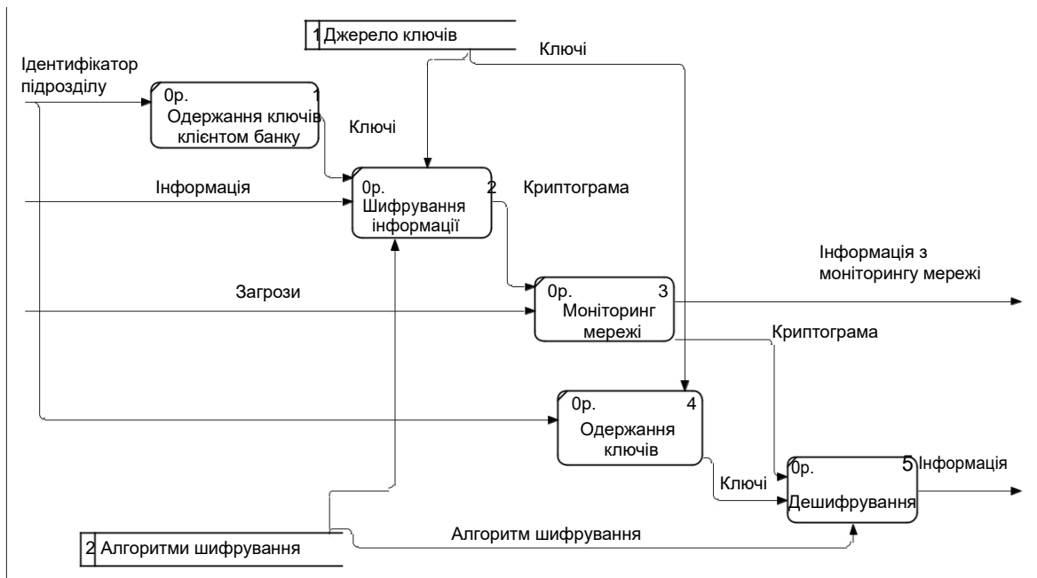
Рис. 1.10. Декомпозиція моделі пасивних атак
